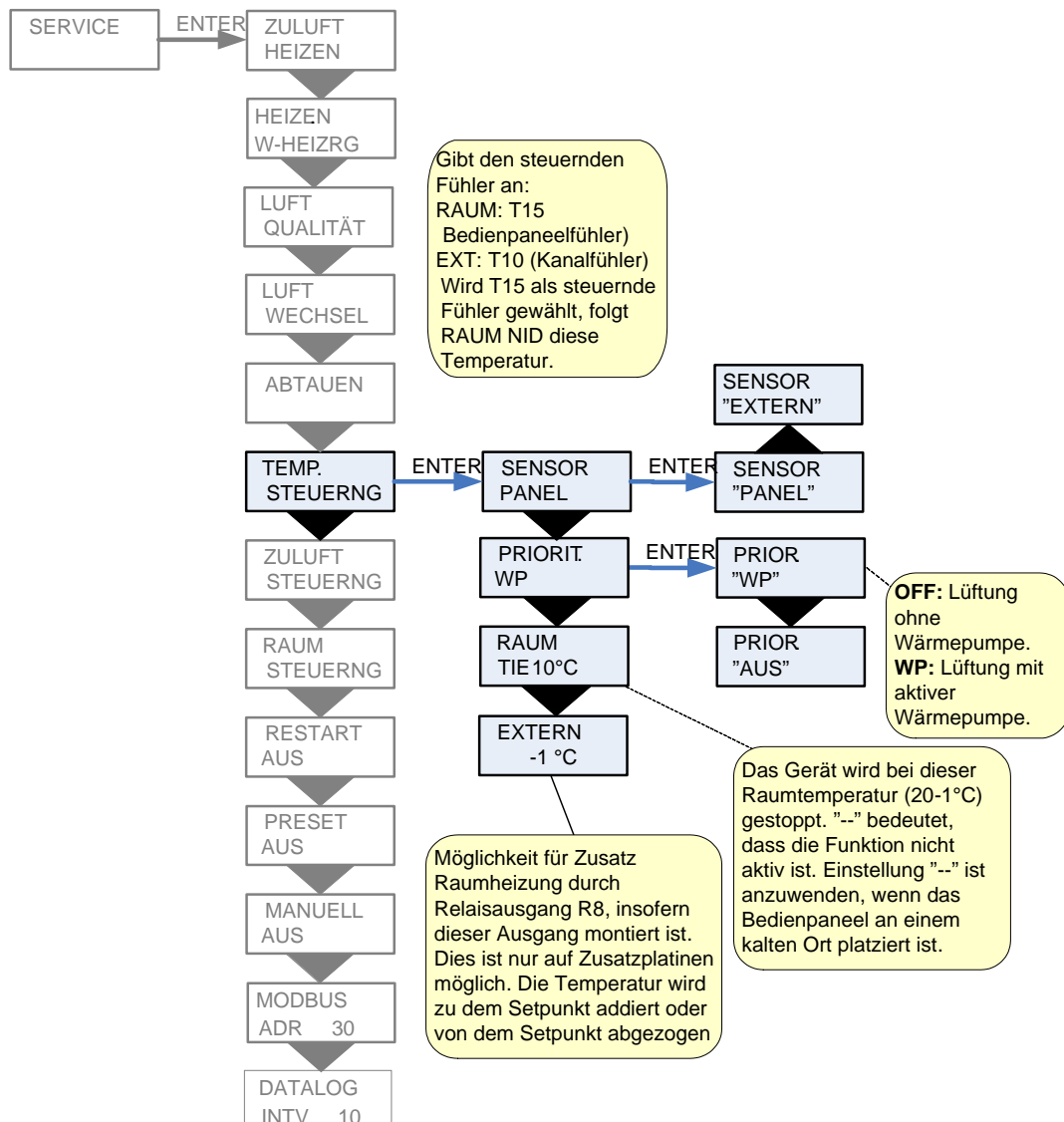
Figur 12: Das Menu " Temp. Steuerung"
