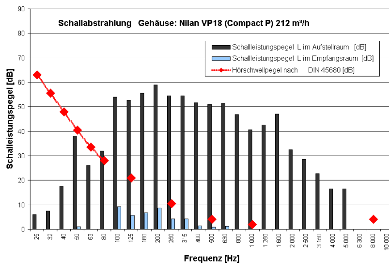
Abbildung 1: Schallabstrahlung des Gehäuses bei Volumenstrom 212 m 3 /h
